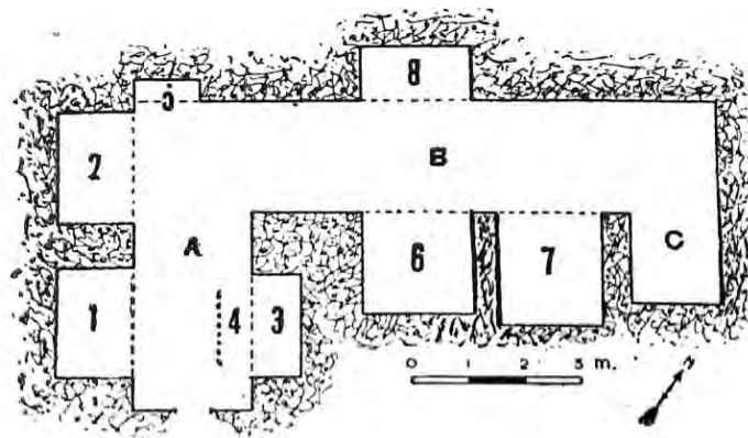
Fig. 18 - Sito 1. Ipogeo Lauridia. Pianta (da Frenkel 1934: 190).
