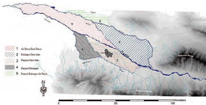
Fig. 5 – Principali canali artificiali nella media valle dello Zeravšān. (© Università degli Studi di Bologna).
