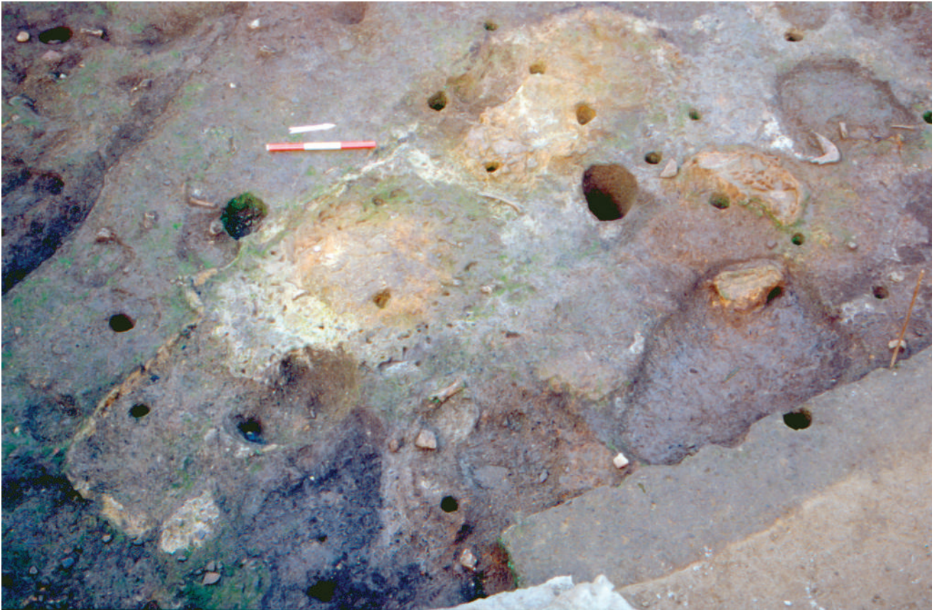
Fig. 53 – Area con strutture di combustione (struttura 7) per la lavorazione del bronzo.
