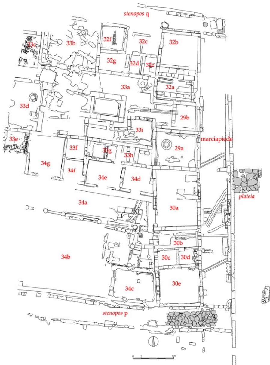
Fig. 2 - Planimetria dell'isolato a nord delle Terme del Foro (rilievi a cura della missione dell'Università degli Studi di Napoli "L'Orientale" e degli Architetti Calcagno e Associati)
